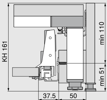
Potreba miesta v korpuse
