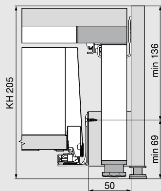
Potreba miesta v korpuse
