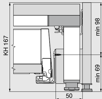
Potreba miesta v korpuse
