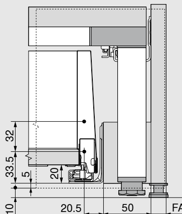
Rozmery osadenia čela pri montáži naskrutkovaním
