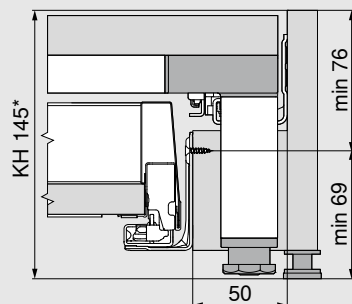
Potreba miesta v korpuse
