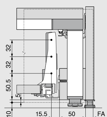
Rozmery osadenia čela pri montáži naskrutkovaním
