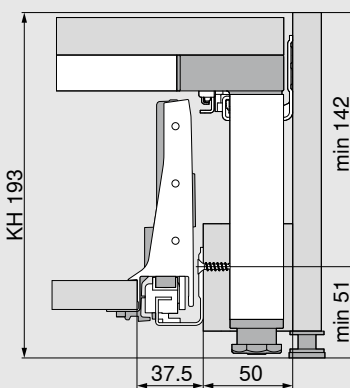
Необходимое пространство в корпусе
