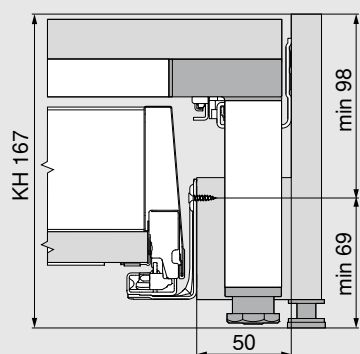
Необходимое пространство в корпусе
