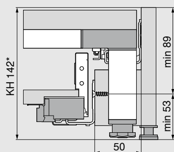
Необходимое пространство в корпусе
