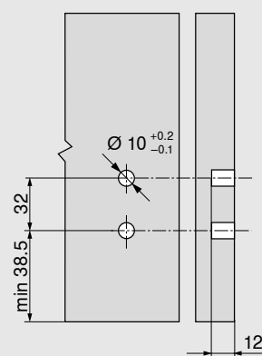
Карта сверления фасада – EXPANDO
