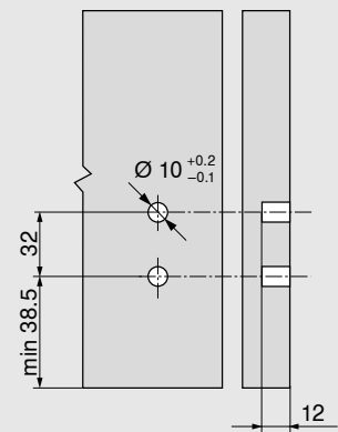
Boormaten front voor EXPANDO
