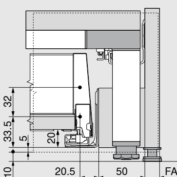
Esipaneeli mõõdud kruvikinnituse puhul
