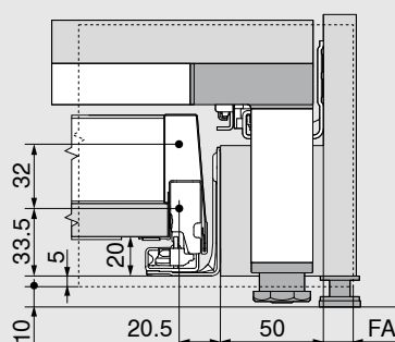
Esipaneeli mõõdud kruvikinnituse puhul
