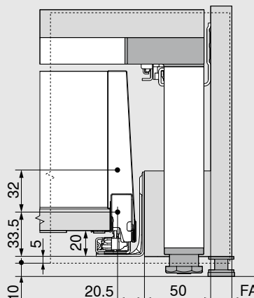
Esipaneeli mõõdud kruvikinnituse puhul
