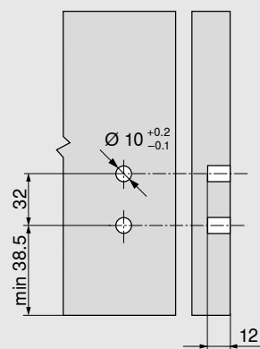
Esipaneeli puurimiskaugus EXPANDO jaoks
