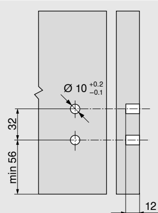
Einbohrmaße Front für EXPANDO
