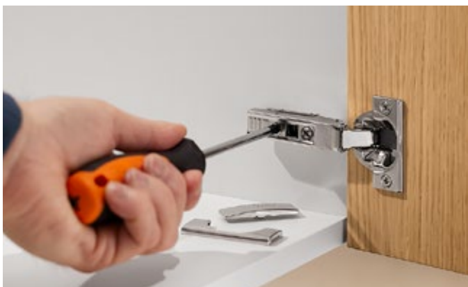
3-dimenzionalno podešavanje fronta, bestepeno podešavanje po dubini preko navojnog puža
