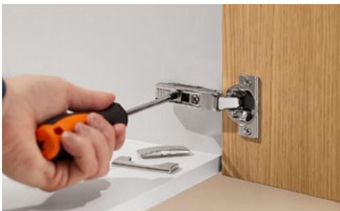
Tridimenzionalna nastavitev sprednje stranice, brezstopenjska nastavitev globine z navojnim polžem
