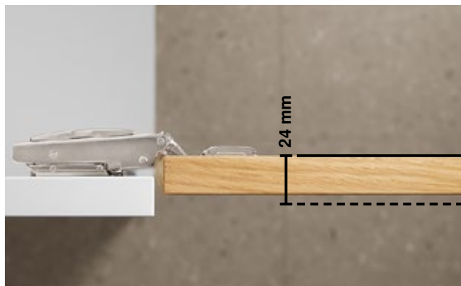
Primeren za debelino sprednje stranice do pribl. 24 mm
