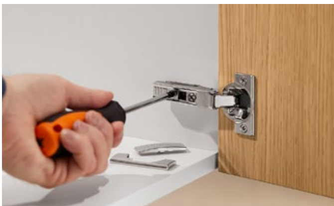
Reglare frontală pe trei dimensiuni, reglare continuă a adâncimii prin șurub elicoidal
