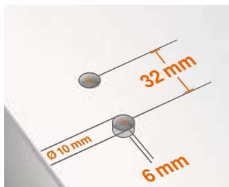
Montering utan grytborrning
