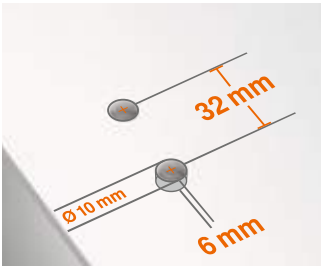
Montagem sem furação do caneco
