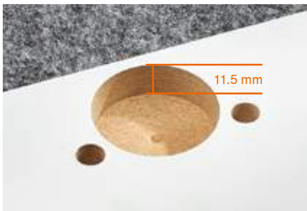
Za lonac šarke je dovoljna dubina bušenja od 11.5 mm.
