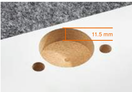
Hingekulbi jaoks piisab puuravast sügavusega 11.5 mm.
