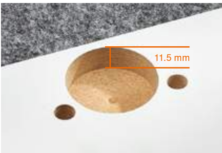
Pro miskú závěsu stačí hloubka vrtání 11.5 mm.
