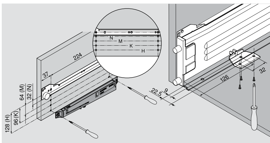
System 32: Montering av BLUMOTION-enheten sker i 32-mm borrhål.
